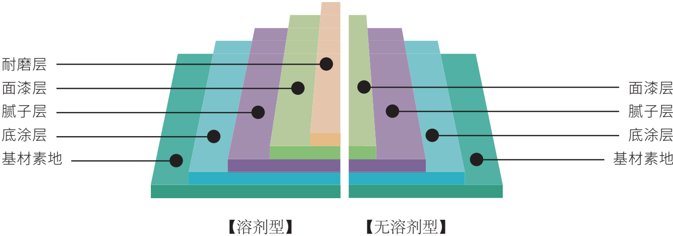
施工剖面图：
