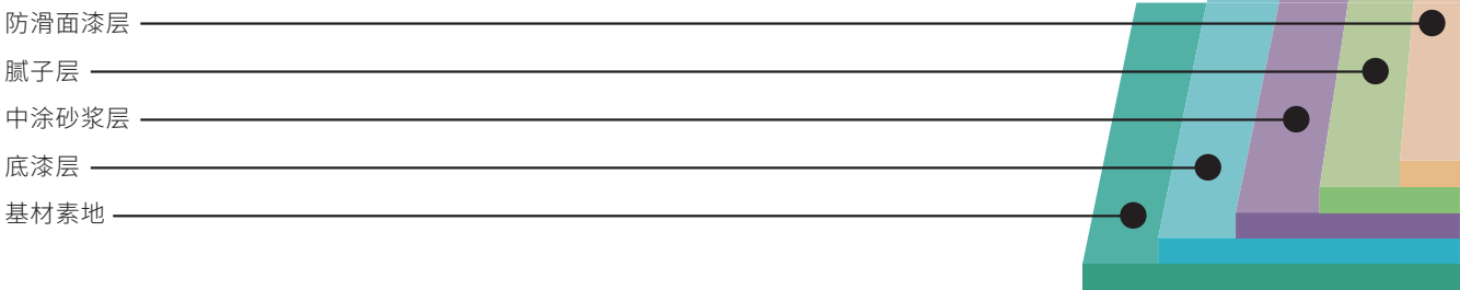
施工剖面图：
