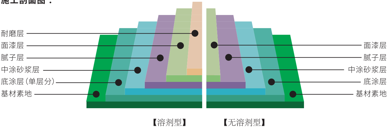
施工剖面图：
